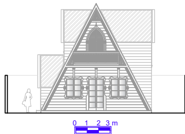
Elevation 01
